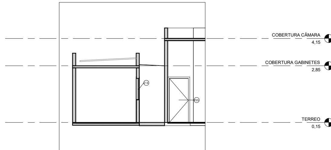
4 Corte 2 1 : 50
