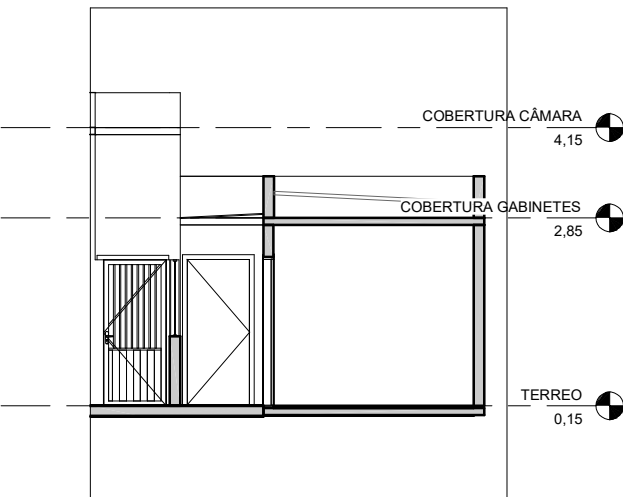
3 Corte 1 1 : 50
